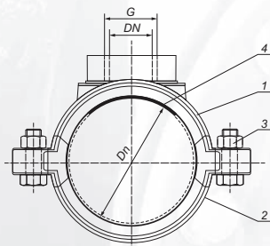
Obejma NOBW z gwintem wewnętrznym
