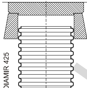
Pokrywa żelbetowa 425 Pierścień żelbetowy 425
