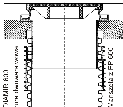
Właz żeliwny 600 Adapter teleskopowy 600 Pierścień żelbetowy odciążający 600
