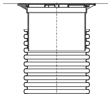
Właz teleskopowy z PP 600
