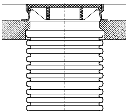
Właz żeliwny 600 Pierścień żelbetowy odciążający 600
